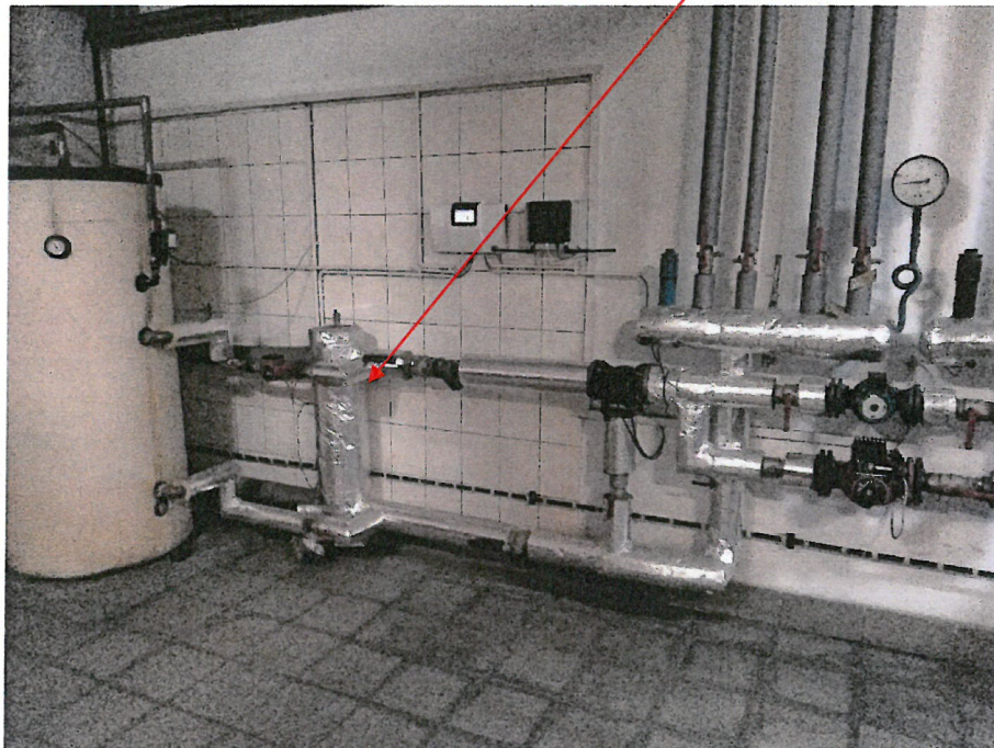
Zdjęcie 5. Sprzęgło hydrauliczne
